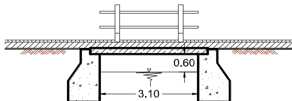
POTONGAN MEMANJANG
