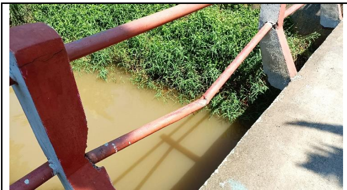
SANDARAN HORIZONTAL BENGGOK
